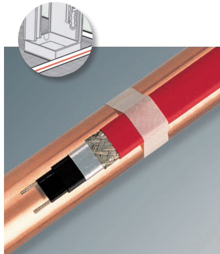
Das Temperaturhalteband wird unmittelbar auf der Rohrleitung verlegt.
